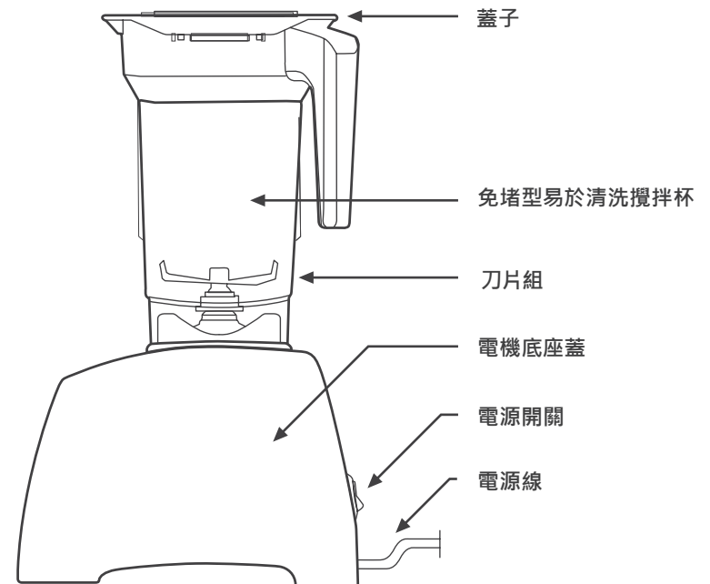
圖2：電機底座和攪拌杯組件側視圖
