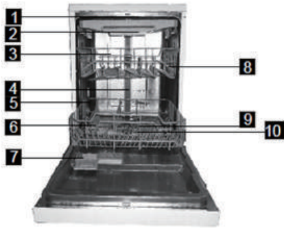
正視圖
